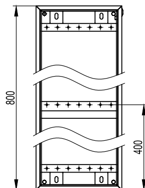
Вигляд спереду Front view
