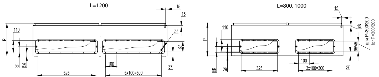
Вид знизу Bottom view
