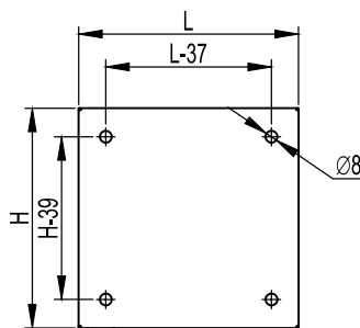
Вигляд ззаду Rear view
