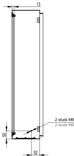
Вид A-A View A-A
