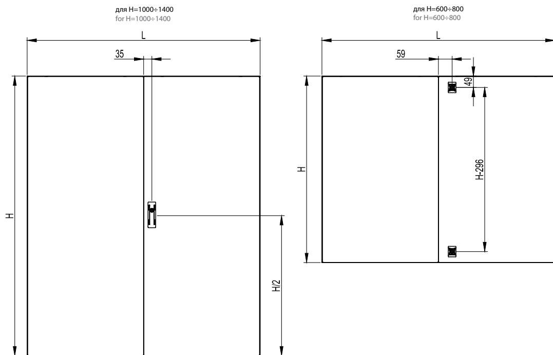
Вид спереду з дверима Front view with door
