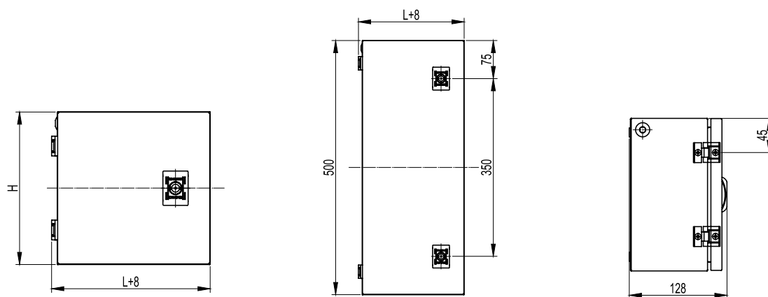
Вигляд спереду Front view
