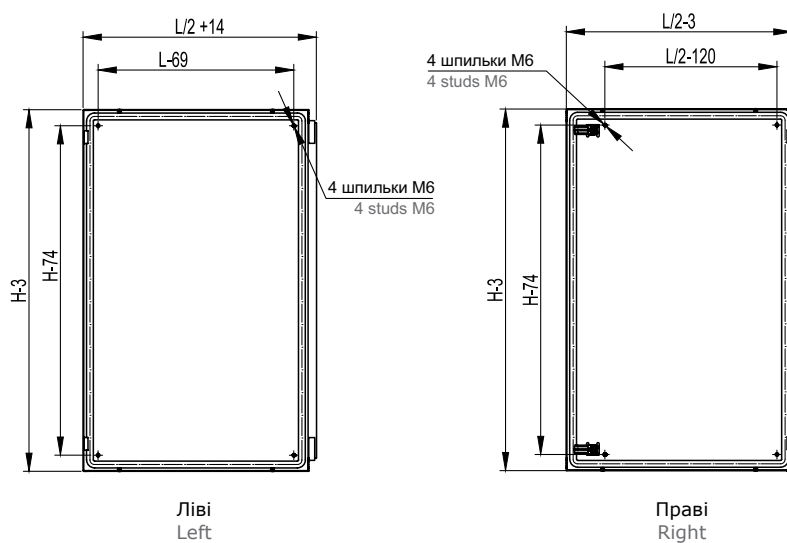
Вигляд дверей зсередини Inside view of door
