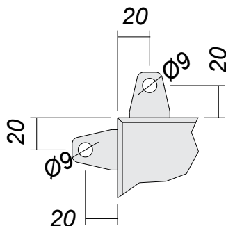
Приклад встановлення кронштейна R5A62 Example of R5A62 bracket installation
