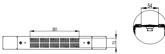
Вигляд спереду Front view
