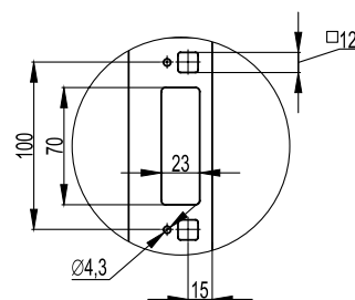
Вигляд A View A
