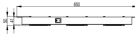
Вигляд спереду Front view
