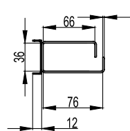
Вигляд збоку Side view
