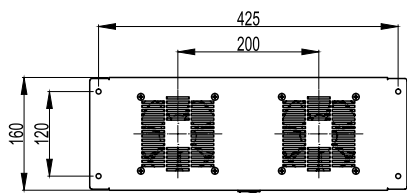
Вигляд зверху Top view
