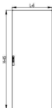
Вигляд спереду Front view
