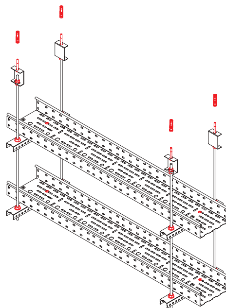
Мал. 2. Приклад конструкції для прокладки кабелю в металевому лотку типу стеля (на двох рівнях). Figure 2. An example of a design for laying a cable in a metal ceiling-type tray (on two levels).
