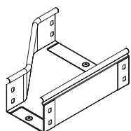
ПЕРЕХІДНИК ЛІВОБІЧНИЙ RRS LEFT-SIDE ADAPTER RRS
