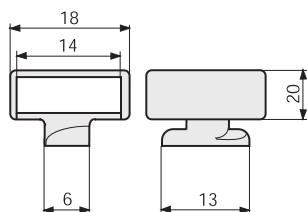
Фіксатор ZP2 ZP2 clamper
