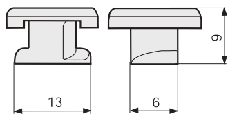
Фіксатор ZP1 ZP1 clamper
